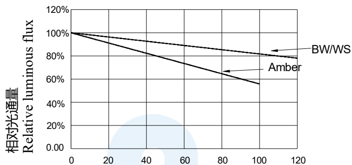
焊盘温度 (T=25°C) Pad temperature (T=25°C)
