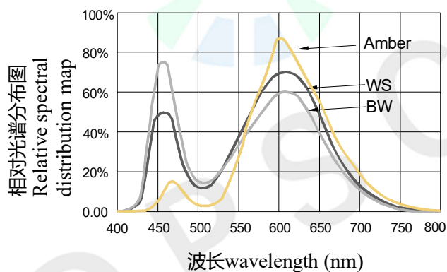
波长特性 Wavelength characteristics
